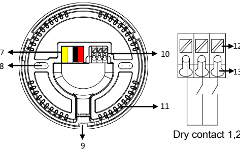
Figure 6. Components - Back View 图 6. 部件 - 背面图
